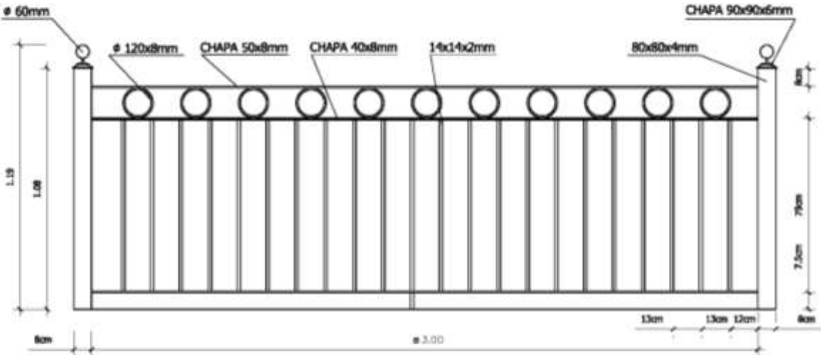
BARANDILLA METALICA MODELO "Avda. Euzkaldierria"
